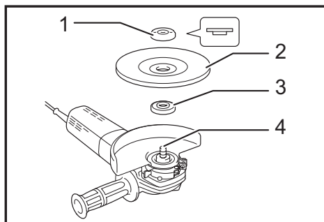
► 1. Contratuera 2. Disco para esmerilar de centro hundido / multidisco 3. Brida interior 4. Eje
