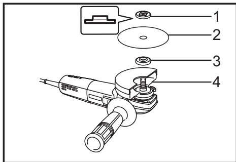
► 1. Contratuera 2. Disco de corte abrasivo / Disco de diamante 3. Brida interior 4. Protector de disco para disco de corte abrasivo / disco de diamante
