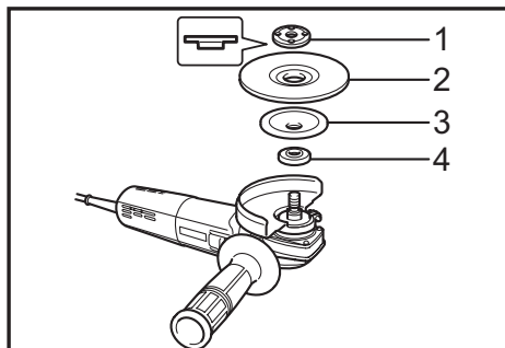
► 1. Contratuera 2. Disco flexible 3. Almohadilla de soporte 4. Brida interior
