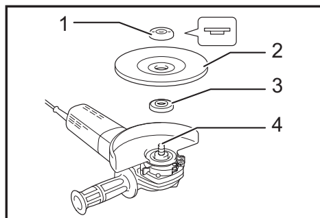
► 1. Contre-écrou 2. Meule à moyeu déporté / Multi-disque 3. Bague interne 4. Axe
